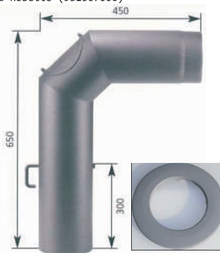
Rauchrohrset inkl. Drosselklappe und Rosette (931507000)
